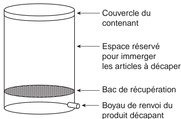
Figure 5.1.11 Bac d'immersion
